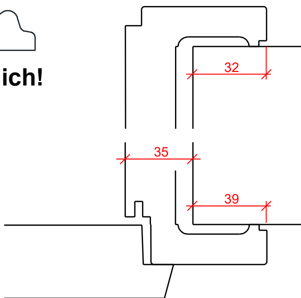
Verkleidungen norm ohne Deutschstab
