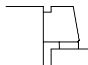
Bei Massivtüren Glasstab norm
