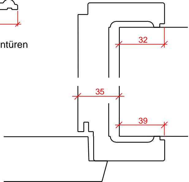
Verkleidungen norm ohne Deutschstab
