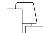
Bei Plattentüren Glasstab überfäلت
